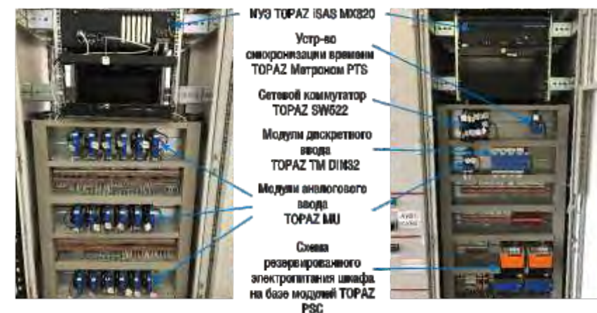
Пример компановки шкафа PAC ПС «Бирюлево» 110 кВ
