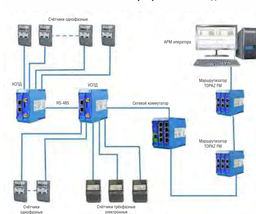
Система АСКУЭ многоквартирного жилого дома
