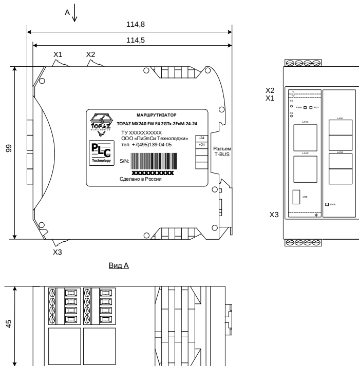
Рисунок В.4 – Габаритные размеры устройств TOPAZ FW MX240 E4 2GTx-2Fxm-2LV, TOPAZ FW MX240 E4 2GTx-2Fxs-2LV
