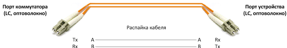
Рисунок 39 – Схема подключения оптоволоконного кабеля
