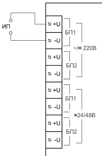
а) Схема подключения питания
