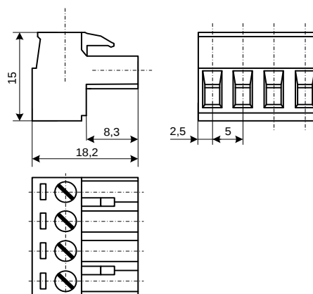
Рисунок 22 – Габаритные размеры разъема MSTBT 2,5/4-ST
