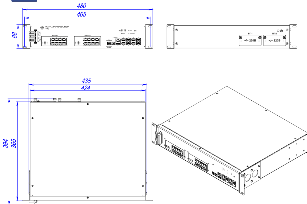
Рисунок В.5 – Габаритные размеры устройств TOPAZ FW MX710
