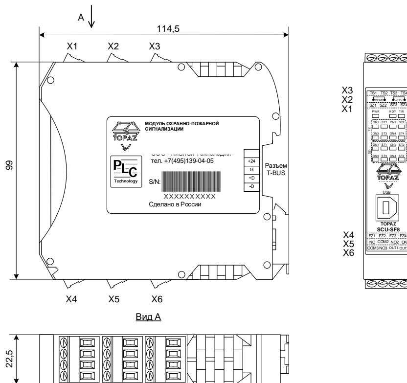
Рисунок А.2 – Габаритные размеры модуля TOPAZ SCU-SF8
