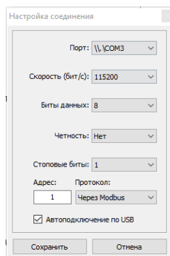
Рисунок 20 – Параметры интерфейсов RS-485 по умолчанию
