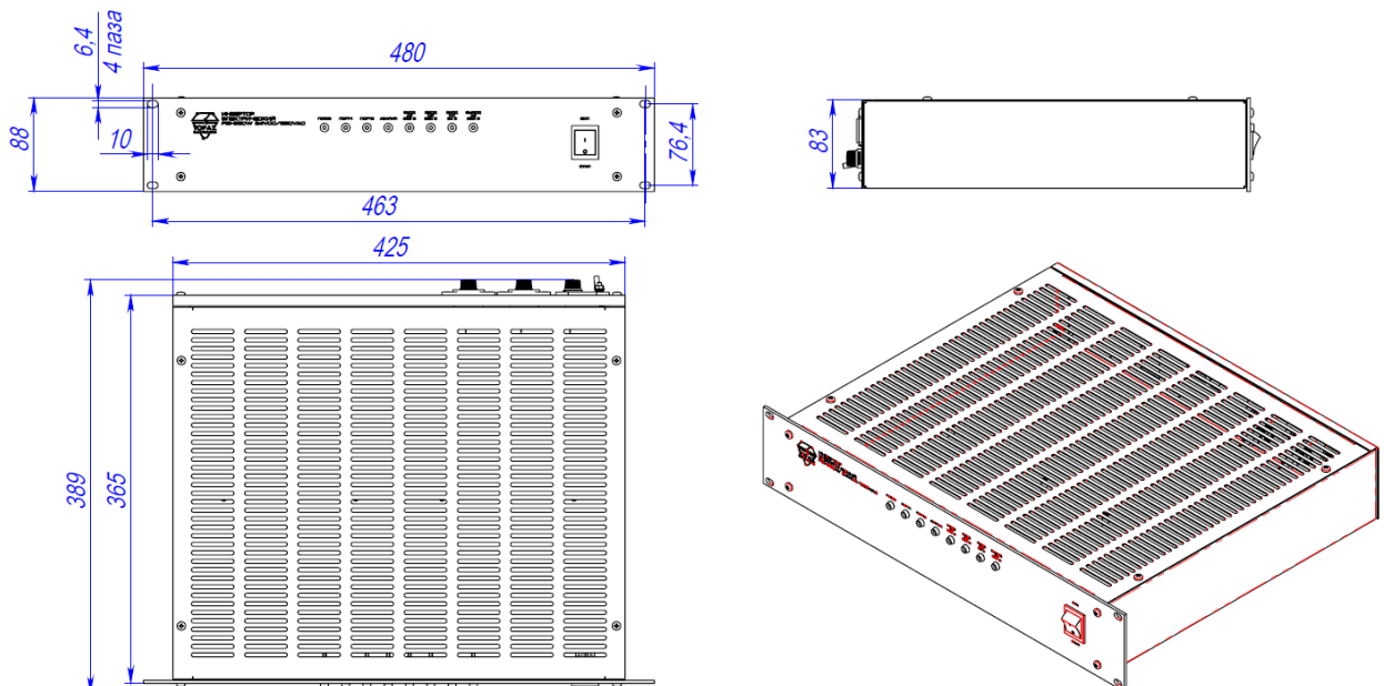
Рисунок 3. Габаритные и установочные размеры устройства
