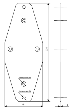
Рисунок 3 – Приспособление для крепления модуля на стене
