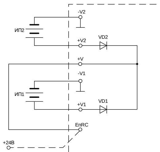
Рисунок 4 – Схема подключения питания
