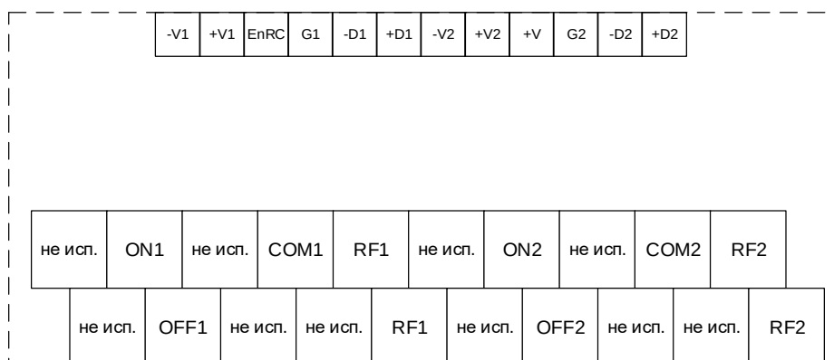
Рисунок А.1 – Назначение клеммных входов модуля TOPAZ MC RTU2 AC/DC5-220V3A-Pr
