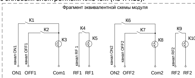
Рисунок 1 – Схема каналов ТУ
