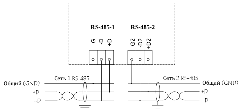
Рисунок 6 – Схема подключения RS-485
