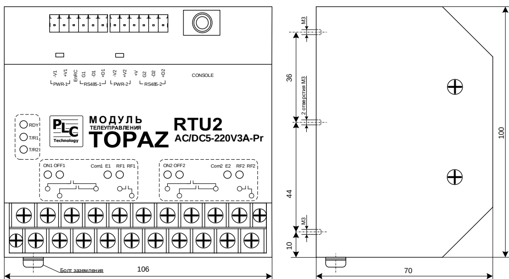
Рисунок А.3 – Габаритные размеры модуля TOPAZ MC RTU2 AC/DC5-220V3A-Pr
