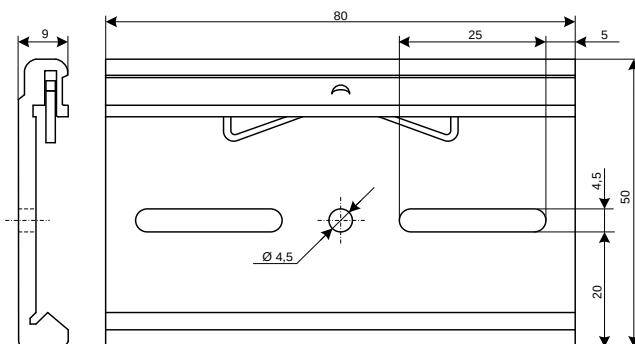
Рисунок 2 – Приспособление для крепления модуля на монтажной рейке
