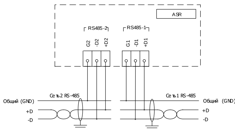
Рисунок 3 – Схема подключения RS-485
