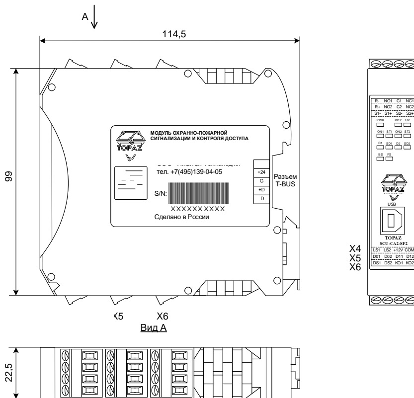
Рисунок А.2 – Габаритные размеры модуля TOPAZ SCU-CA2-SF2
