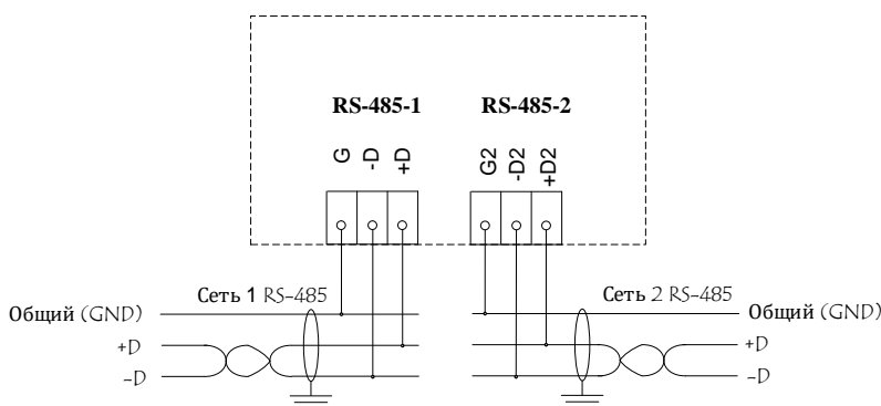
Рисунок 4 – Схема подключения RS-485
