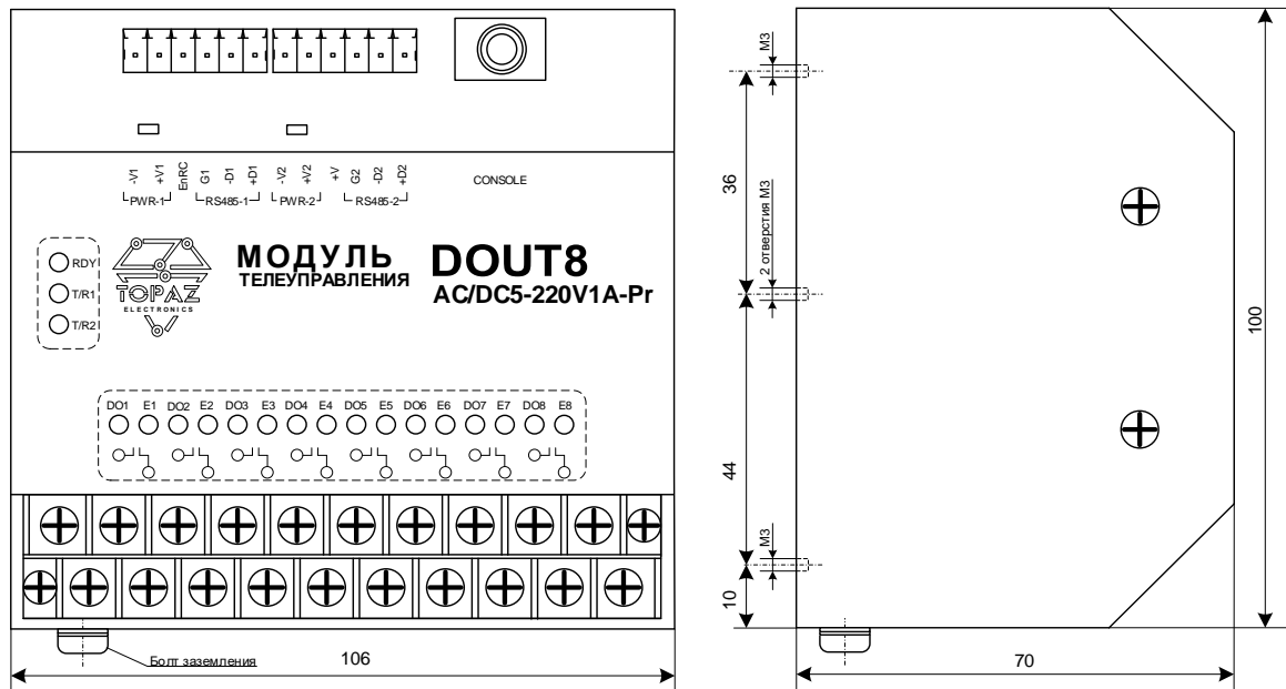
Рисунок А.1 – Габаритные размеры модуля TOPAZ MC DOUT8 AC/DC5-220V1A-Pr
