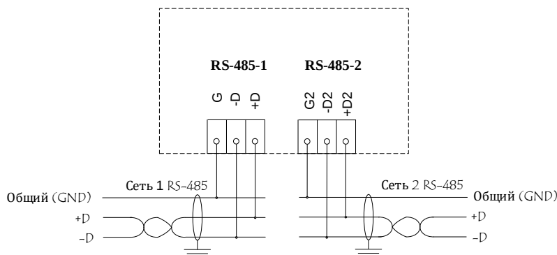
Рисунок 4 – Схема подключения RS-485
