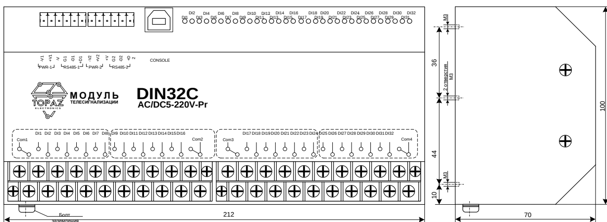
Рисунок А.3 – Габаритные размеры модуля TOPAZ MC DIN32C AC/DC5-220V-Pr
