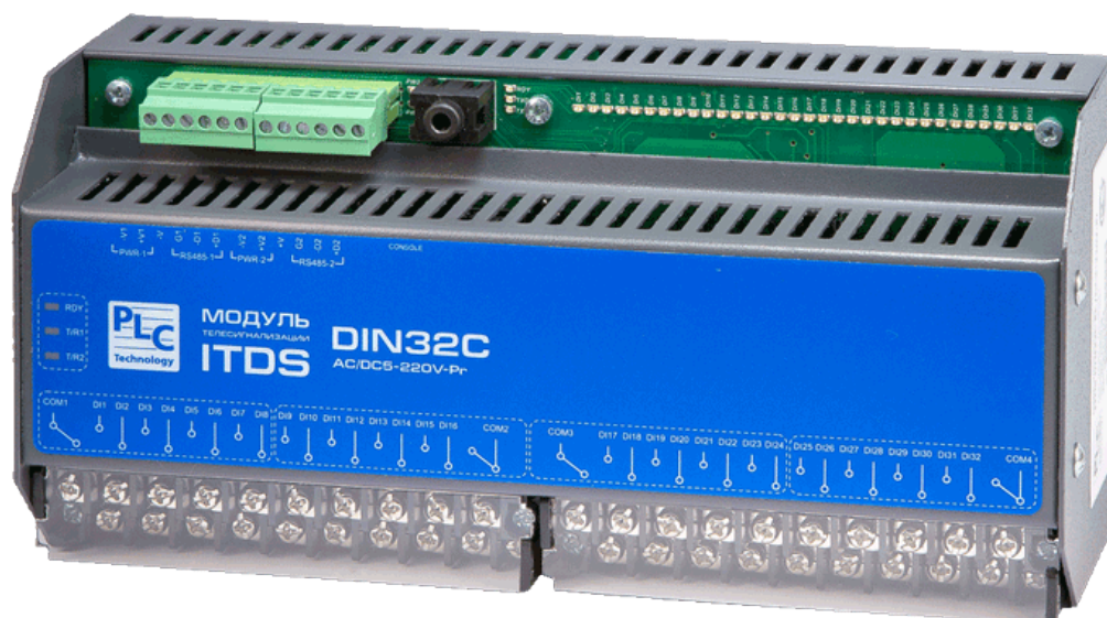
Рисунок А.1 – Внешний вид модуля TOPAZ MC DIN32C AC/DC5-220V-Pr версии 1
