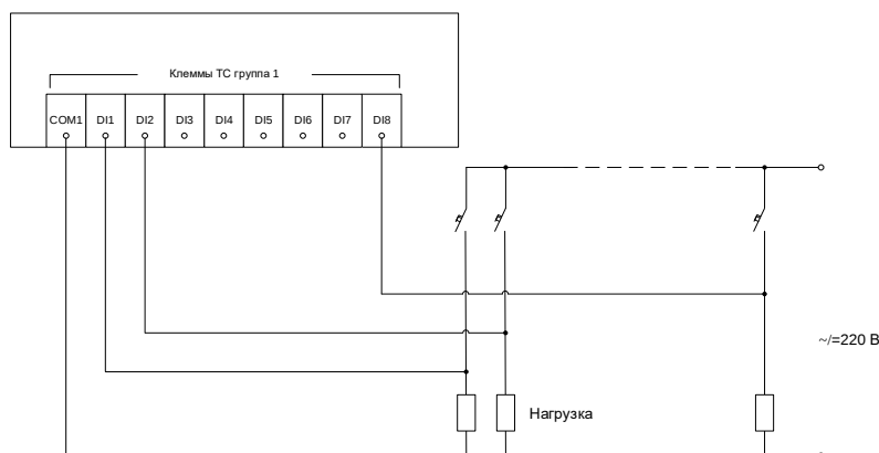
Рисунок 6 – Подключение каналов ТС группы 1 к цепям контроля наличия напряжения
