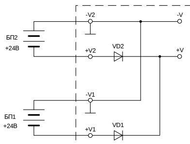
Рисунок 3 – Схема подключения питания
