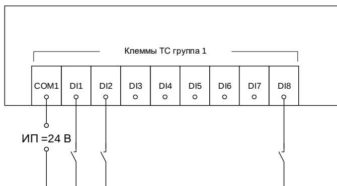
Рисунок 5 – Подключение каналов ТС группы 1
